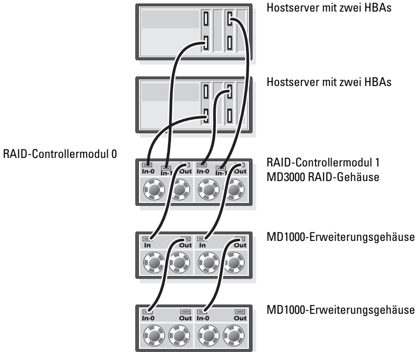
Abbildung 1-4. Direct-Attach SAS-Cluster verkabeln
