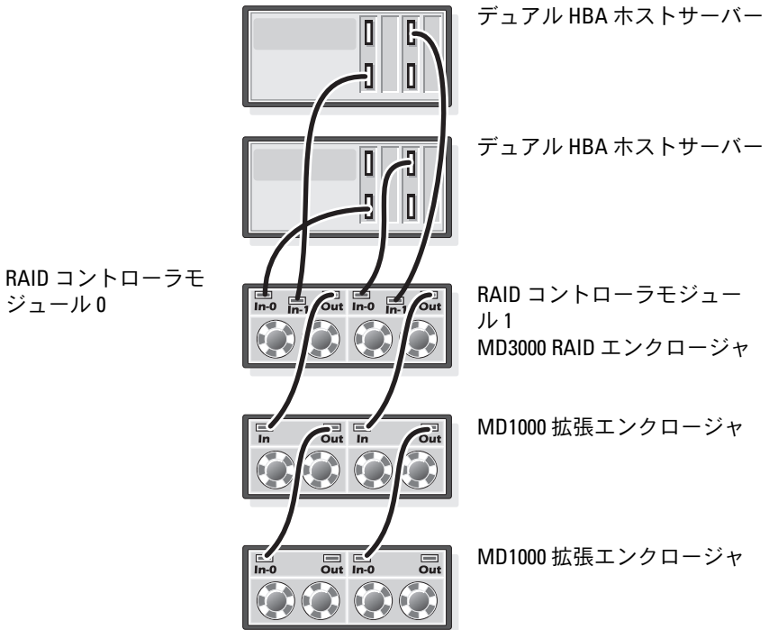
図 1-4. 直接接続 SAS クラスターのケーブル接続
