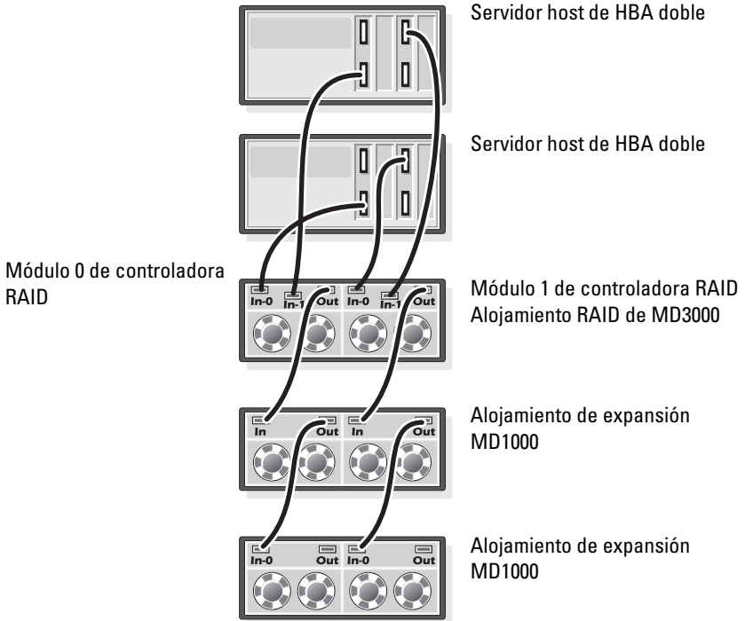
Ilustración 1-4. Cableado de un clúster SAS de conexión directa
