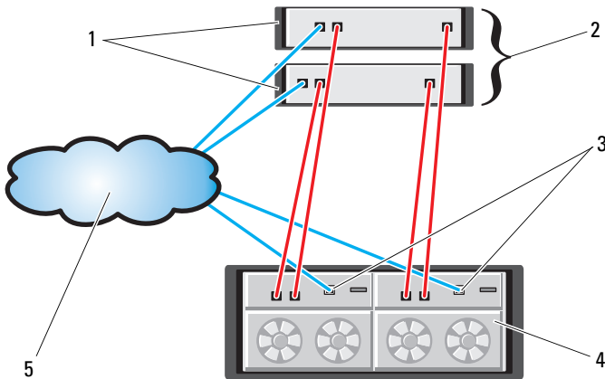
Ilustración 1-5. Cableado de los clústeres iSCSI de conexión directa
