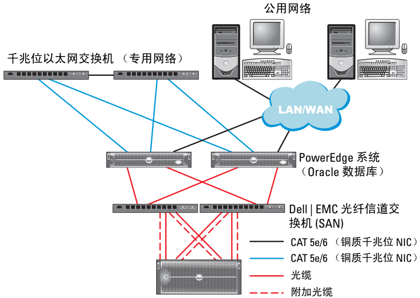
图 1-1. SAN 连接的光纤信道群集的硬件连接
