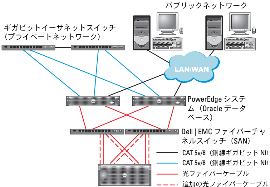
図 1-1. SAN 接続のファイバーチャンネルクラスタ用のハードウェア接続
