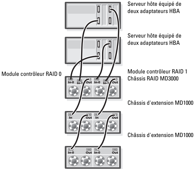
Figure 1-4. Câblage d'un cluster SAS à connexion directe
